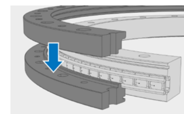
Lager schließen
