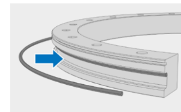
Laufringe einlegen
